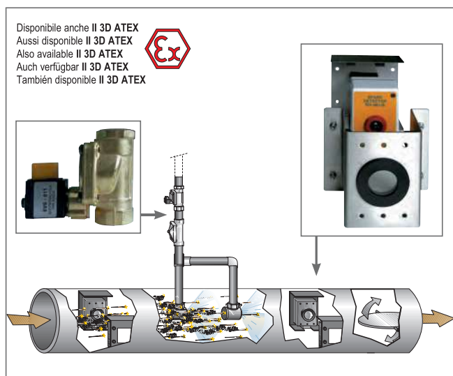
RILEVAMENTO E SPEGNIMENTO SCINTILLA SYSTEME DE DETECTION ET EXTINGUITION D'ÉTINCELLES SPARK DETECTION AND EXTINGUISHING SYSTEM FUNKENERKENNUNGS UND FUNKENLÖSCHUNGS SISTEMA DE RELEVADO Y APAGADO DE CHISPAS
